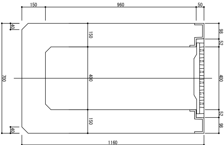
断面図
